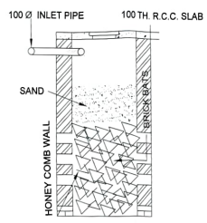
SECTION D-D SCALE: 1:50
